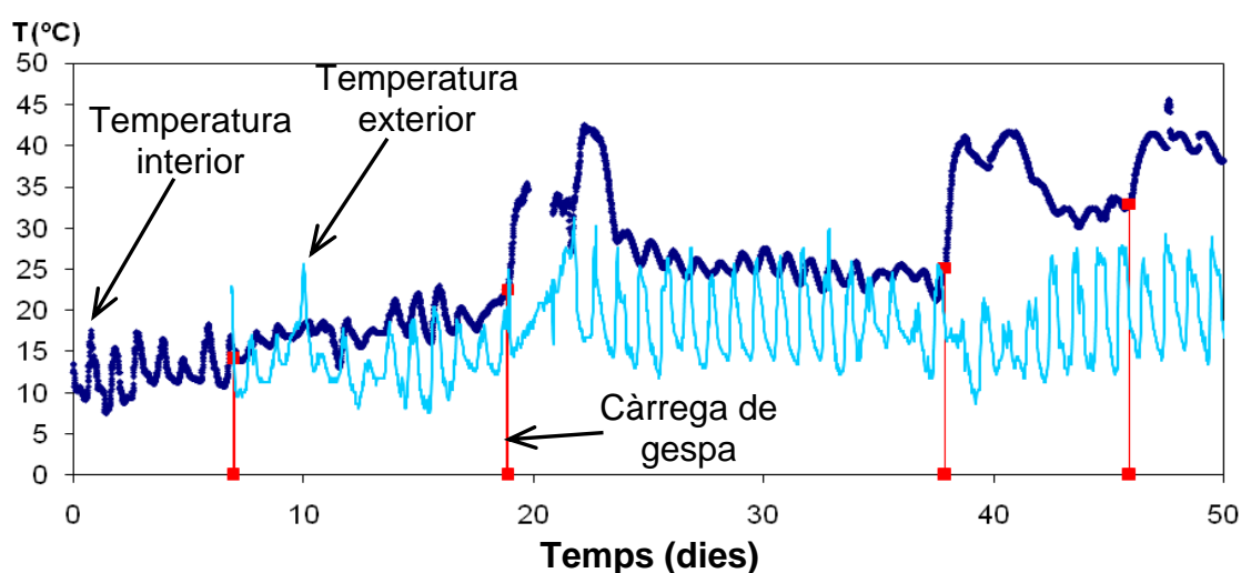
Figura 2. Primers dies d'evolució de la temperatura dins i fora del compostador 400 P. S'indiquen les càrregues de gespa.
